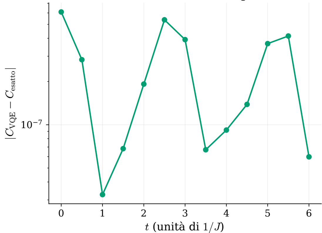
Scostamento (scala log)
