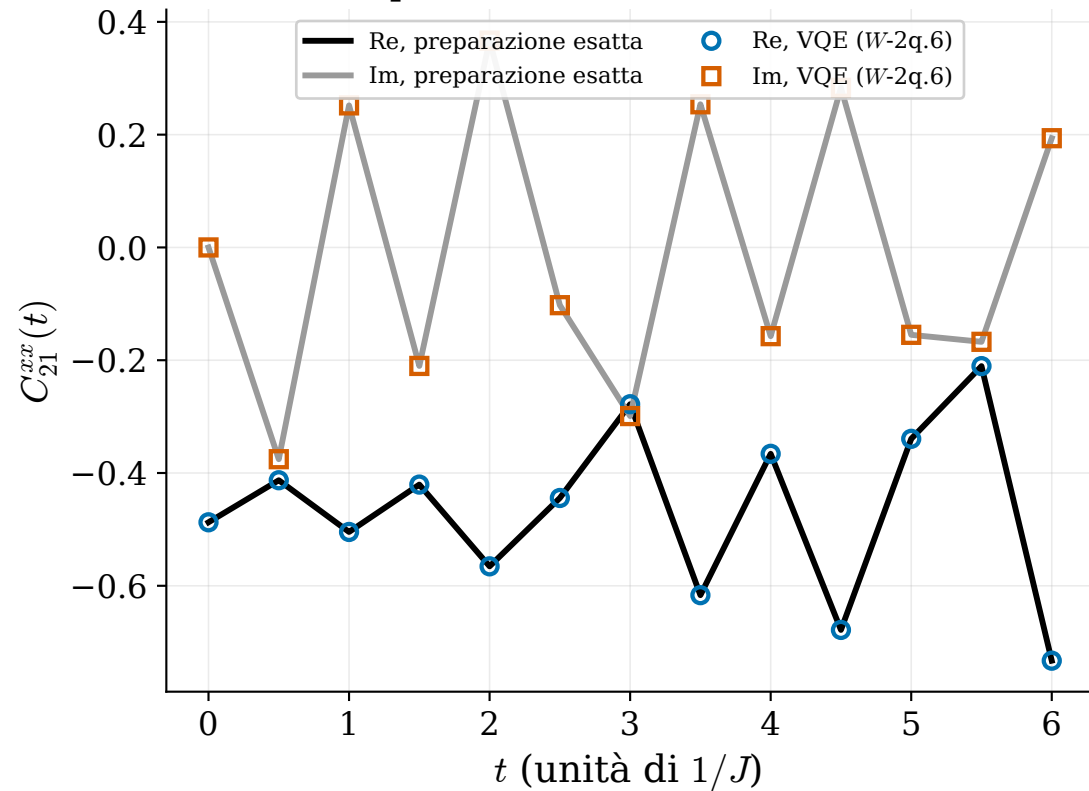
Preparazione esatta contro VQE
